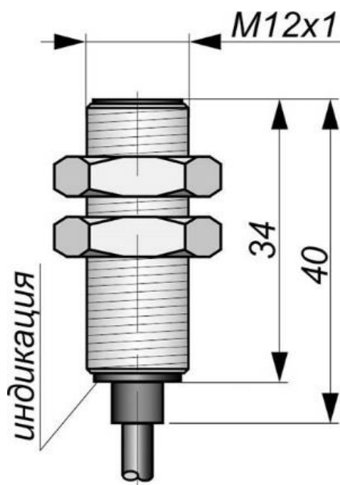
Габаритный чертеж
