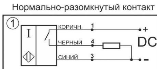
Схема соединения
