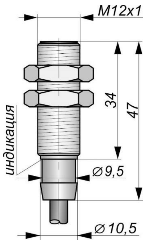
Габаритный чертеж
