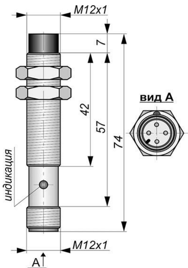
Габаритный чертеж
