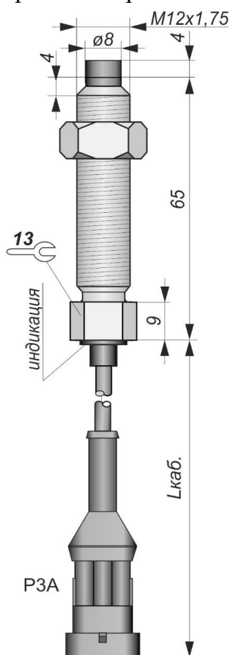
Габаритный чертеж
