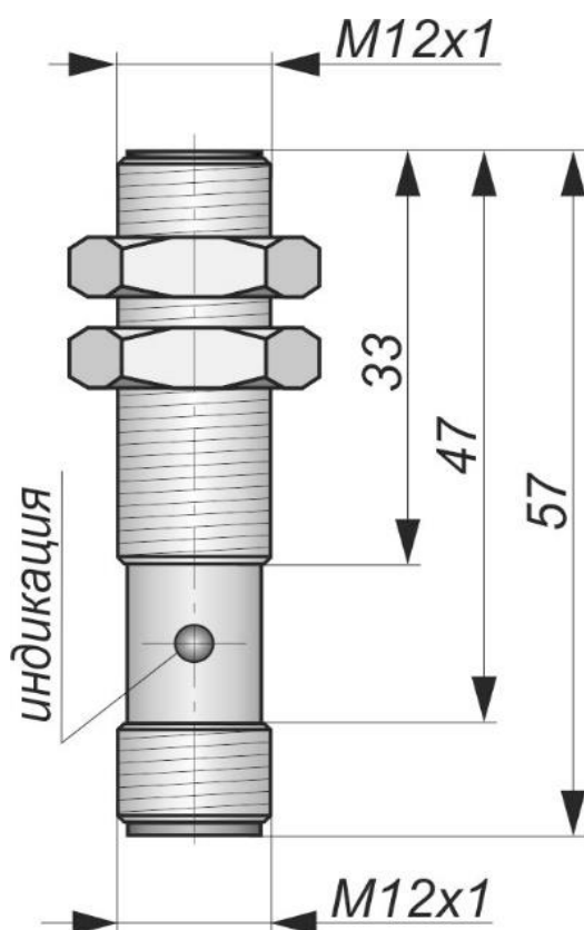
Габаритный чертеж
