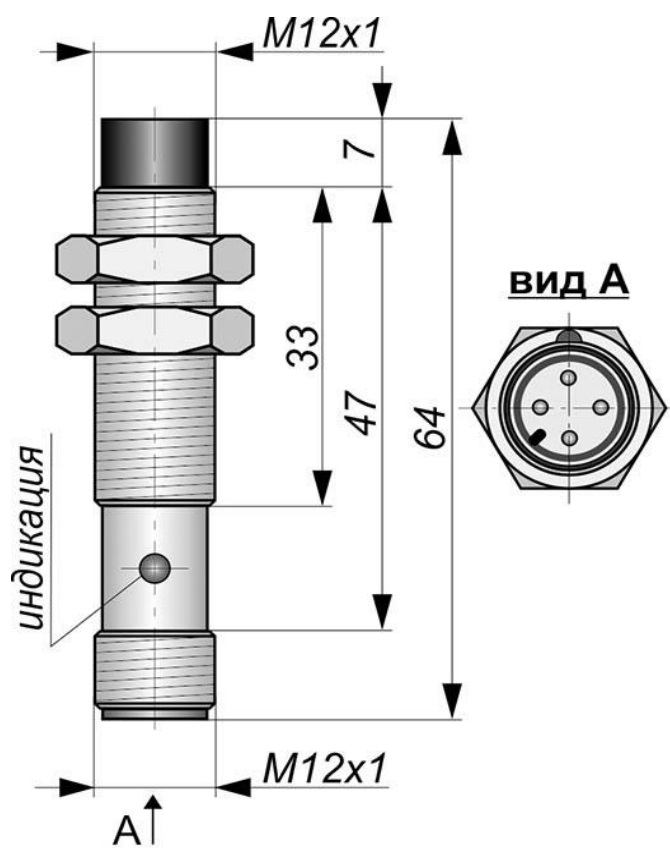
Габаритный чертеж
