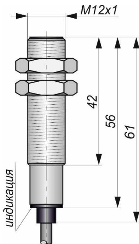
Габаритный чертеж
