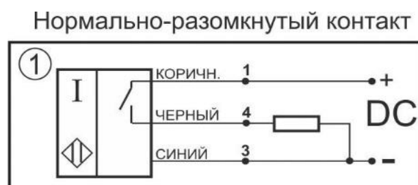
Схема соединения
