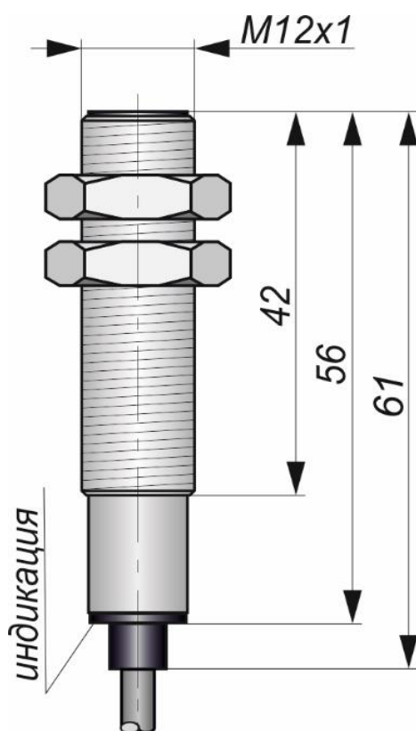
Габаритный чертеж
