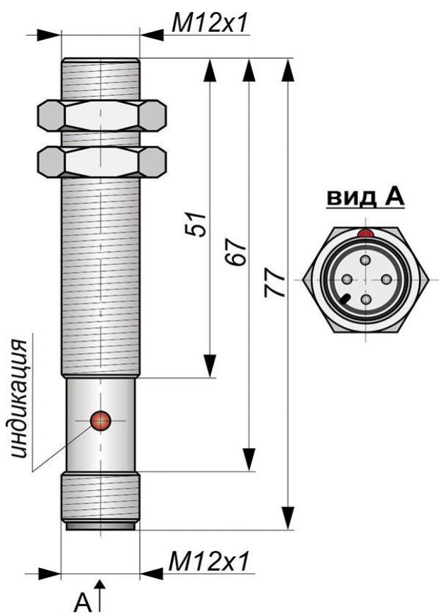
Габаритный чертеж
