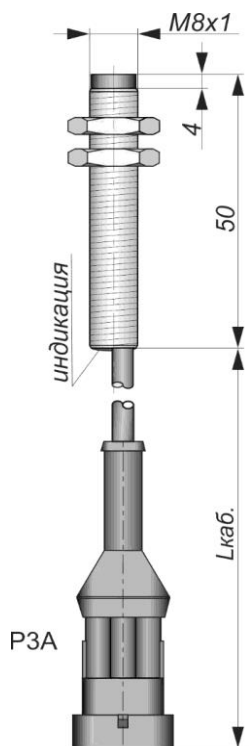
Габаритный чертеж
