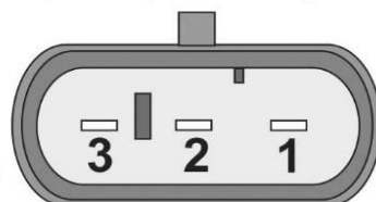
Нормально-разомкнутый контакт
