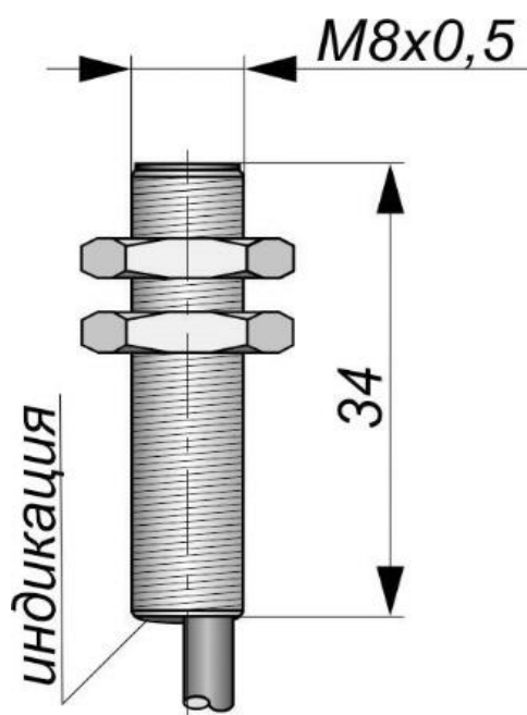
Габаритный чертеж
