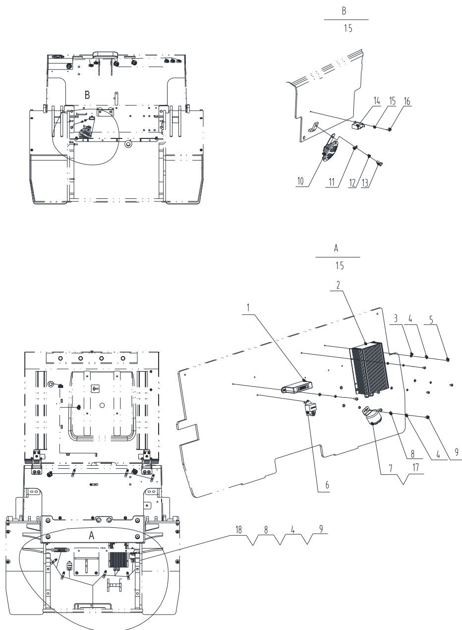
Рис. 82 Электрическая система CPD13, CPD16, CPD18, CPD20, CPD25
