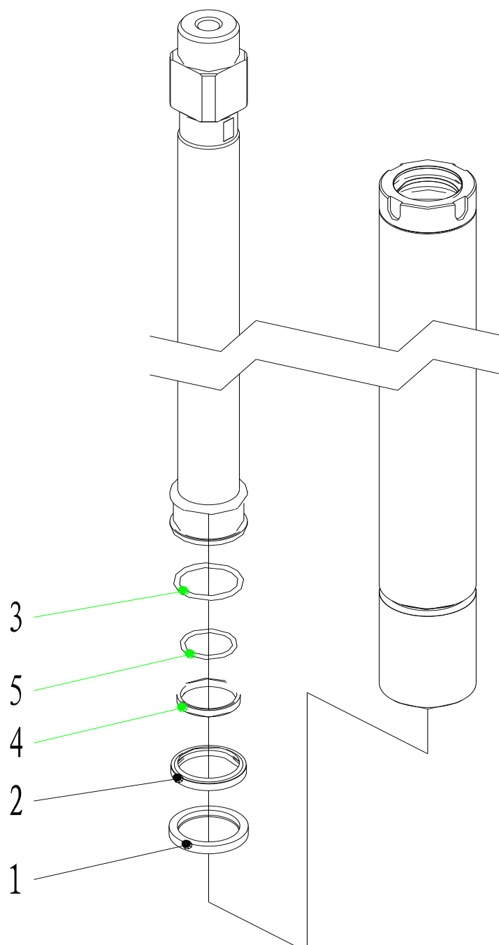
Рис. 105 Задний подъемный цилиндр (CBM2A-A0071)
