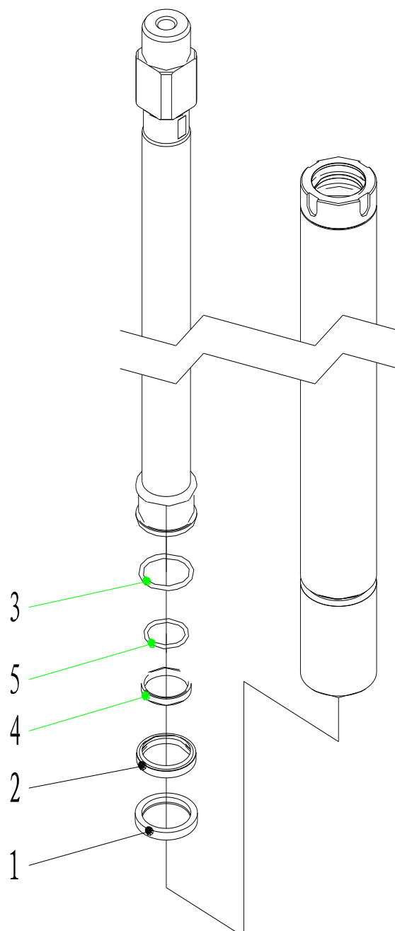
Рис. 114 Задний подъемный цилиндр (ССМ1А-А0071)
