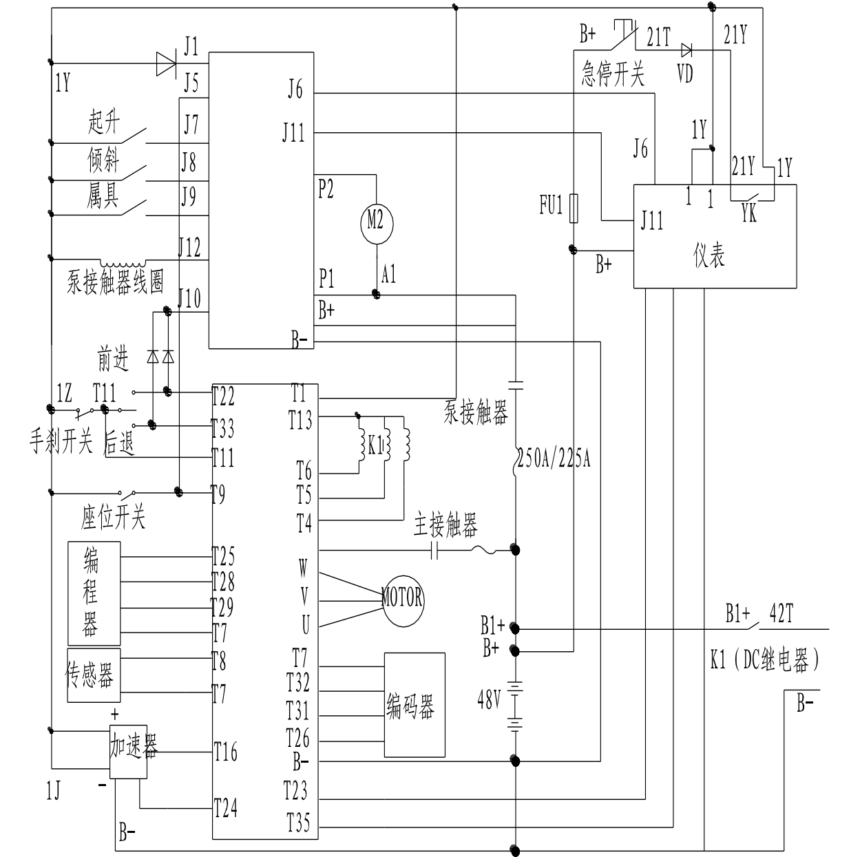
Рис. 63 Электрическая система CPD13, CPD16, CPD18, CPD20, CPD25
