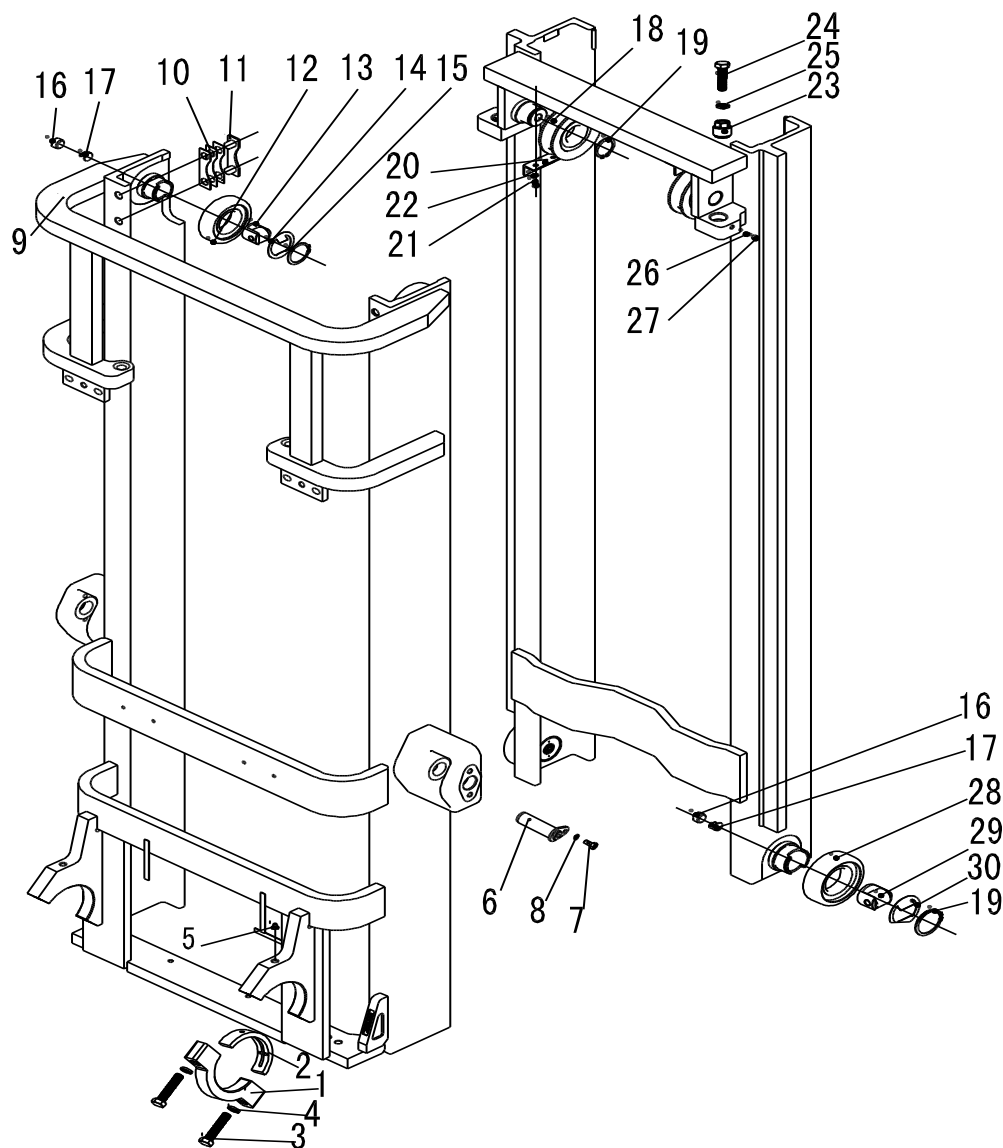
Рис. 95 Мачта ( С2М1А)
