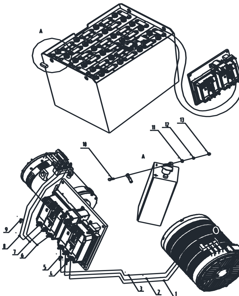
Рис. 61 Электрическая система CPD13, CPD16, CPD18/ CPD20, CPD25
