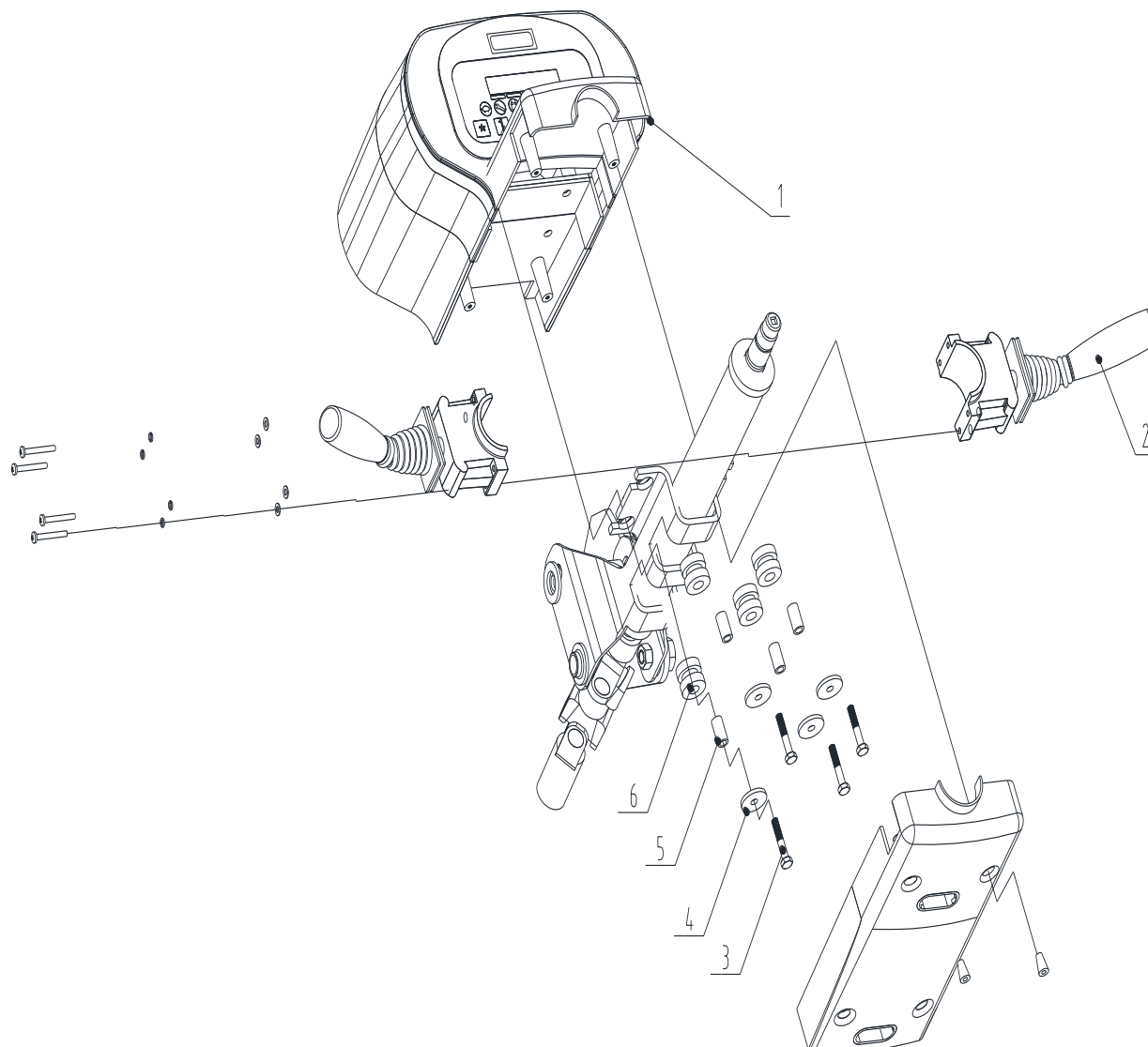
Рис. 59 Электрическая система CPD13, CPD16, CPD18, CPD20, CPD25
