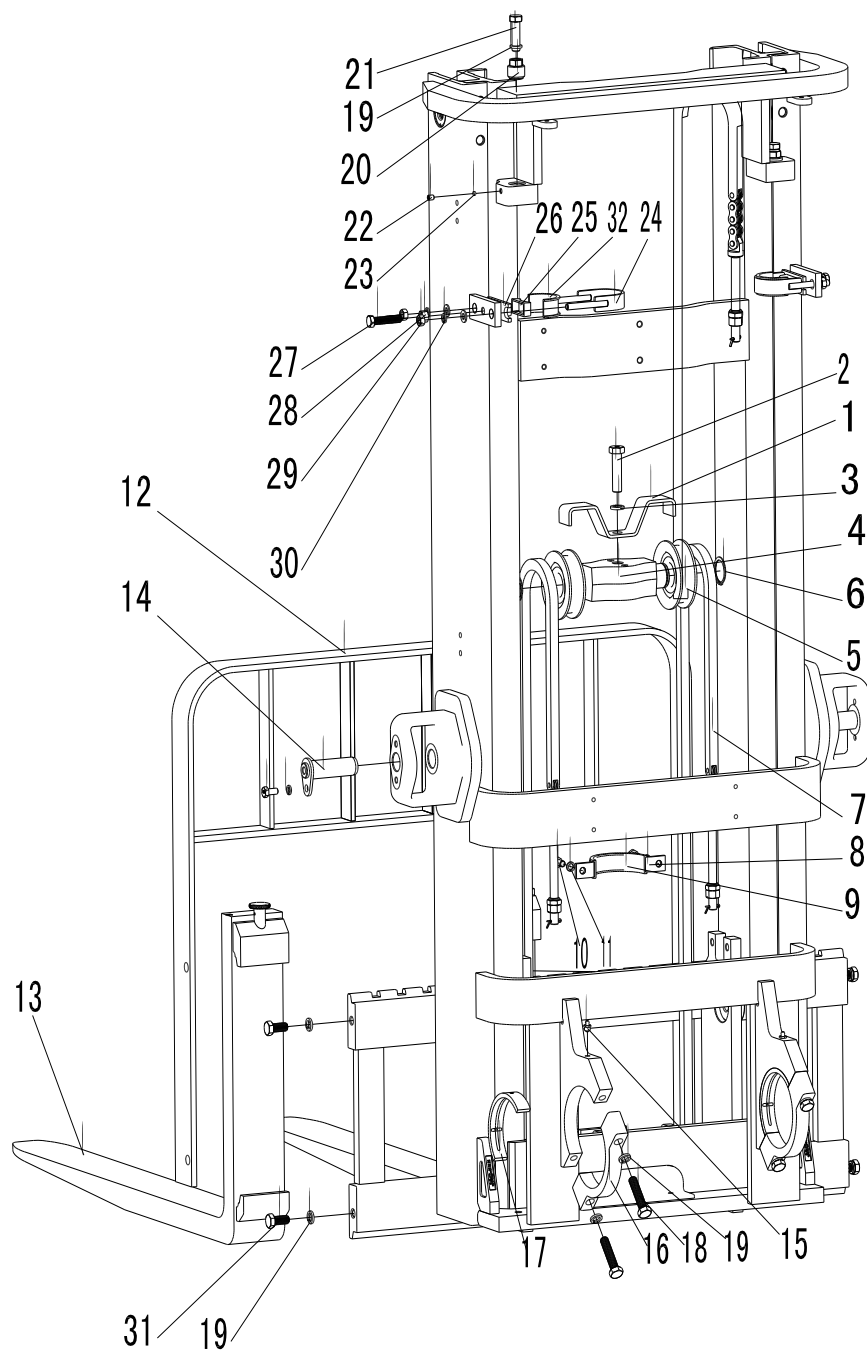
Рис. 100 Мачта (двойная, свободный ход) (СВМ1А)
