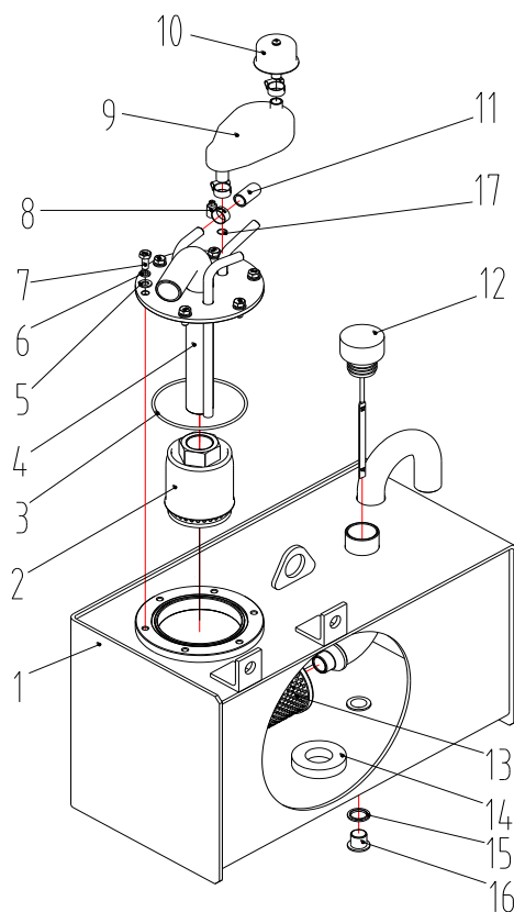
Рис. 93 Гидравлический бак CPD13, CPD16, CPD18/ CPD20, CPD25
