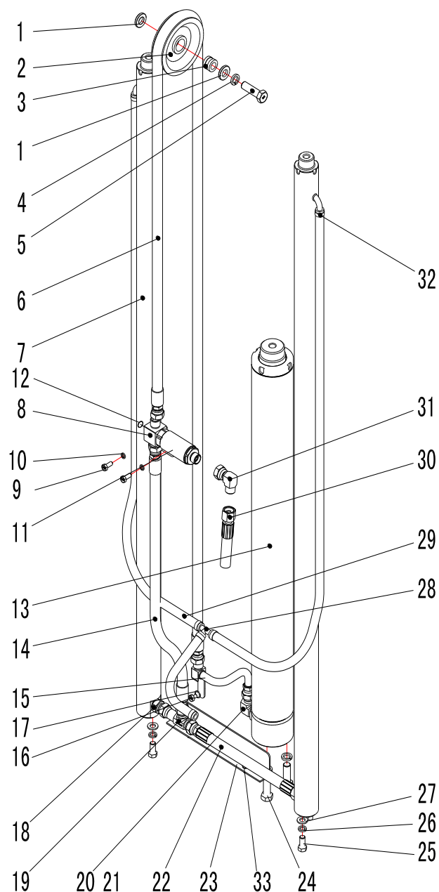
Рис. 113 Гидравлическая система (ССМ1А-18001)
