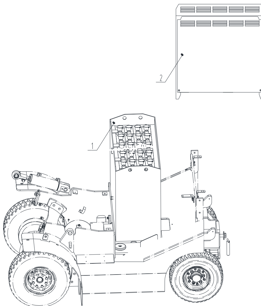
Рис. 49 Электрическая система CPD20, CPD25
