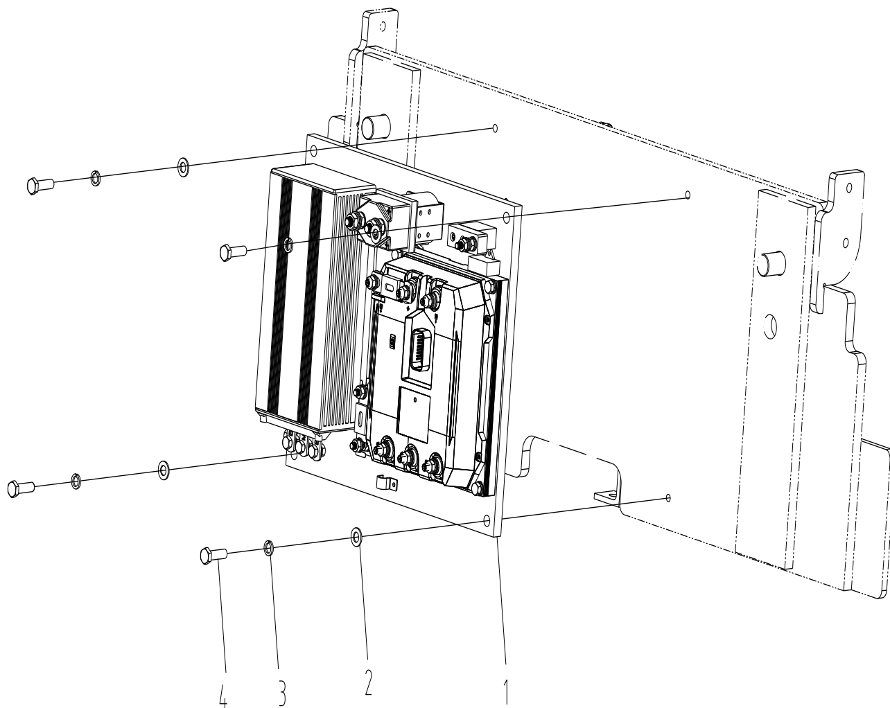
Рис. 64 Электрическая система CPD13, CPD16, CPD18
