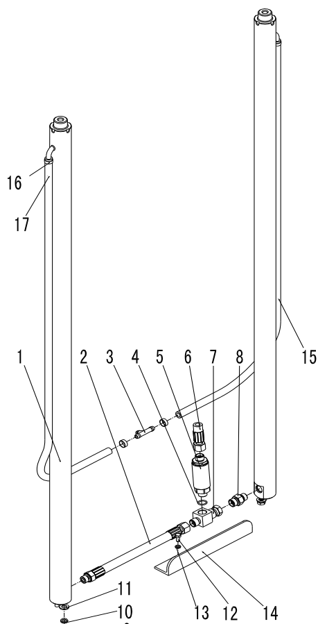
Рис. 97 Гидравлическая система мачты ( C2M1A-13001)
