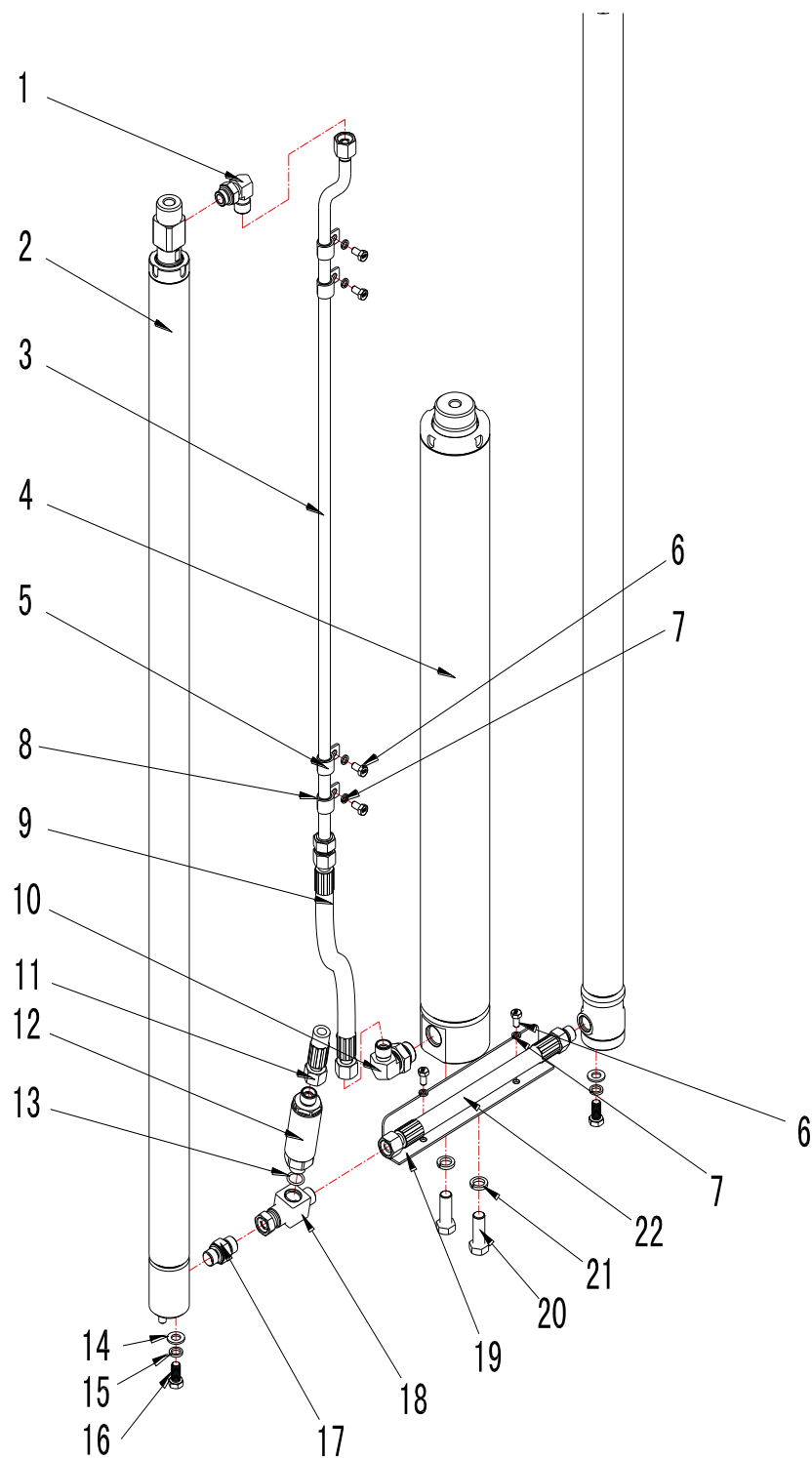
Рис. 104 Гидравлическая система мачты (CBM1A-14001)
