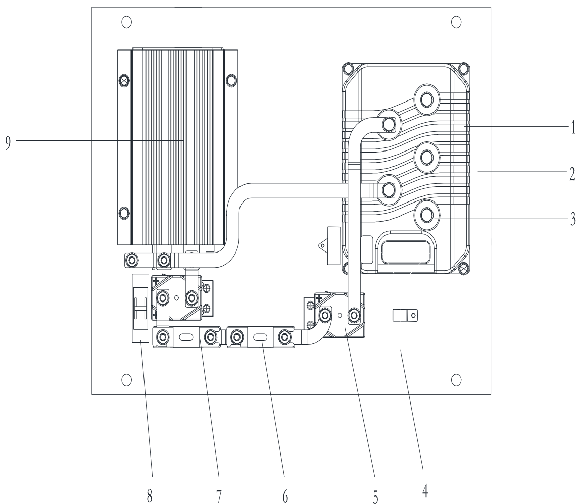
Рис. 66 Электрическая система CPD13, CPD16, CPD18
