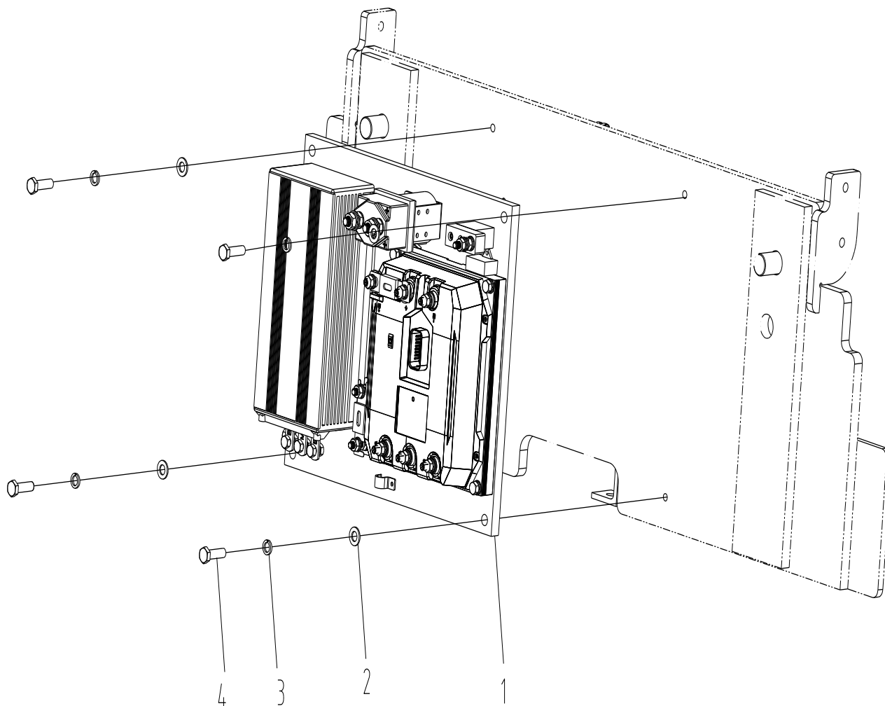
Рис. 37 Электрическая система CPD20, CPD25
