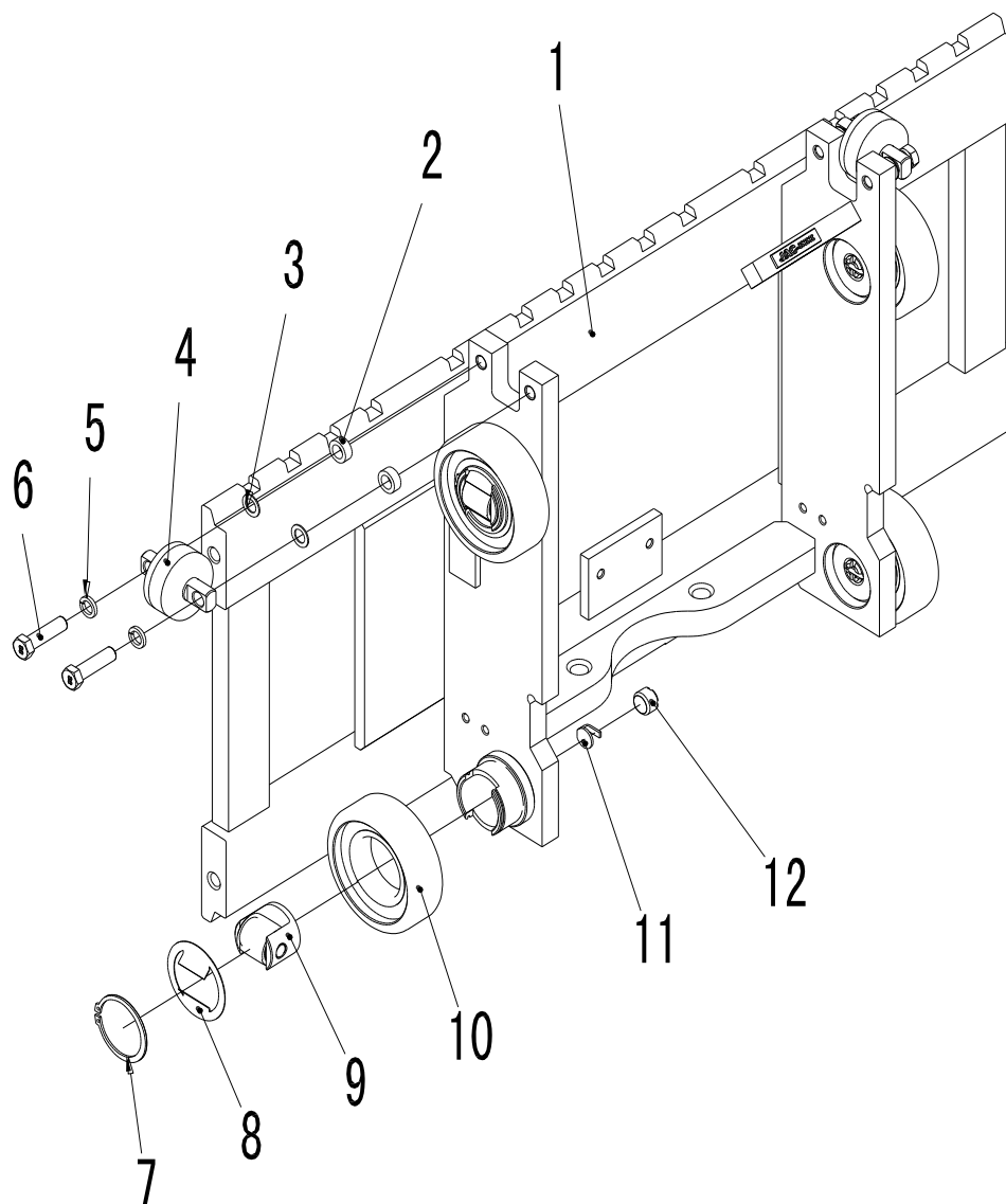
Рис. 103 Установка вилочной рамы(СВМ1А-11001)
