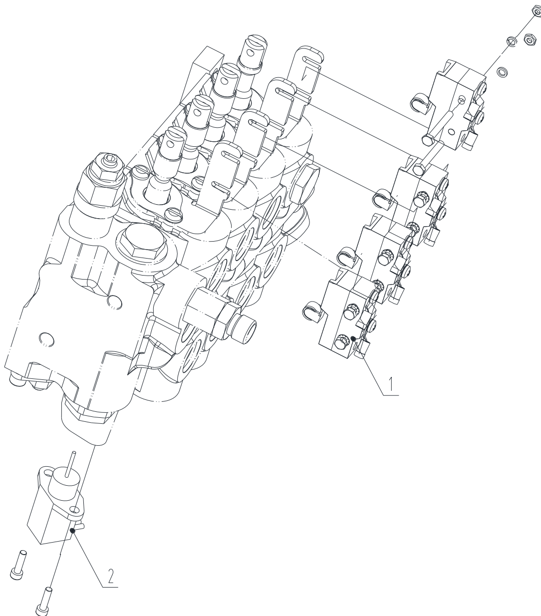
Рис. 86 Электрическая система CPD13, CPD16, CPD18, CPD20, CPD25
