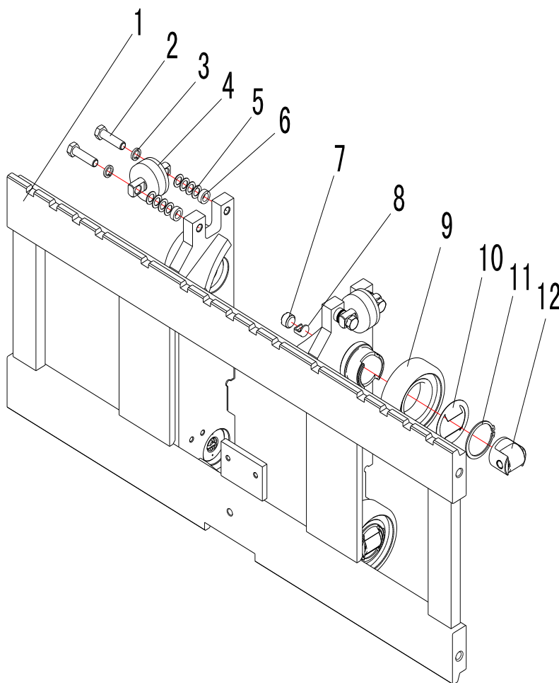
Рис. 112 Установка вилочной рамы (ССМ1А-16001)
