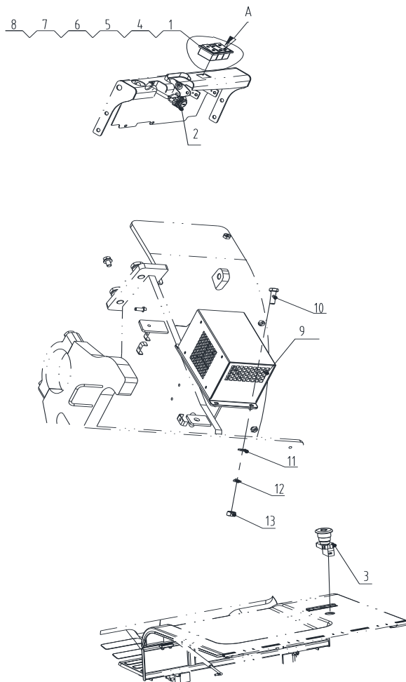
Рис. 56 Электрическая система CPD13, CPD16, CPD18, CPD20, CPD25
