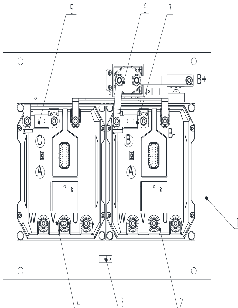
Рис. 39 Электрическая система CPD20, CPD25
