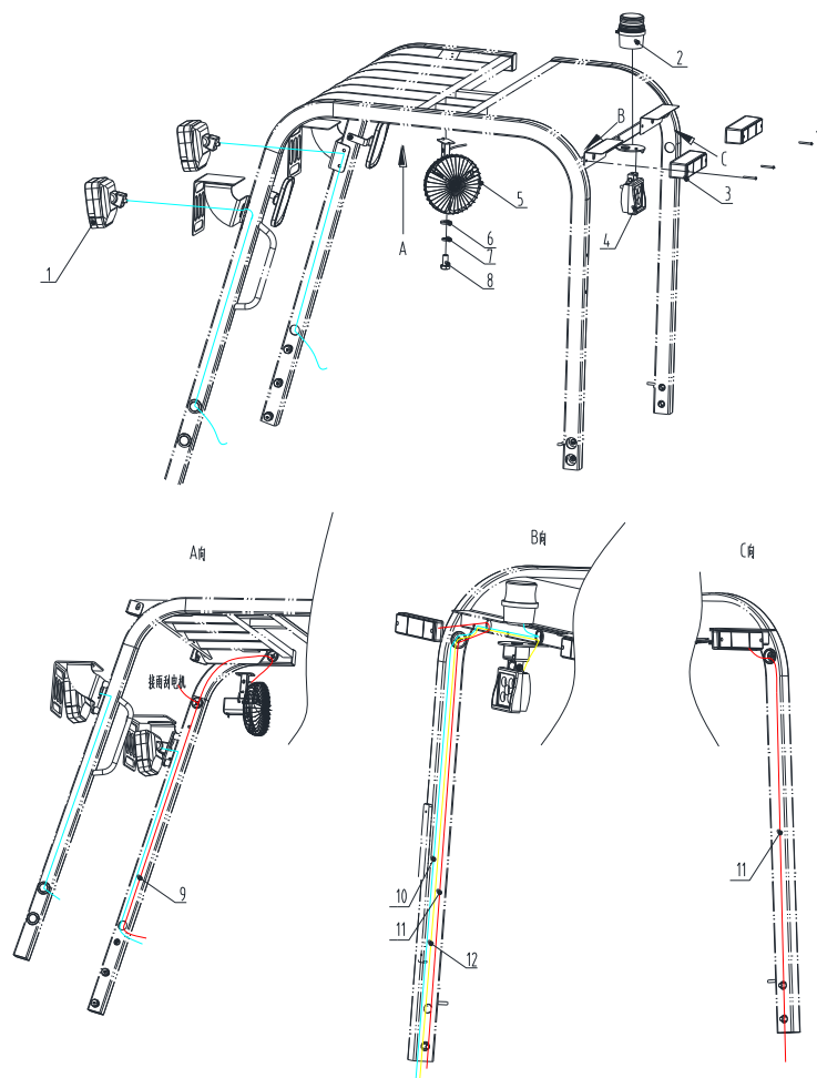
Рис. 81 Электрическая система CPD13, CPD16, CPD18, CPD20, CPD25
