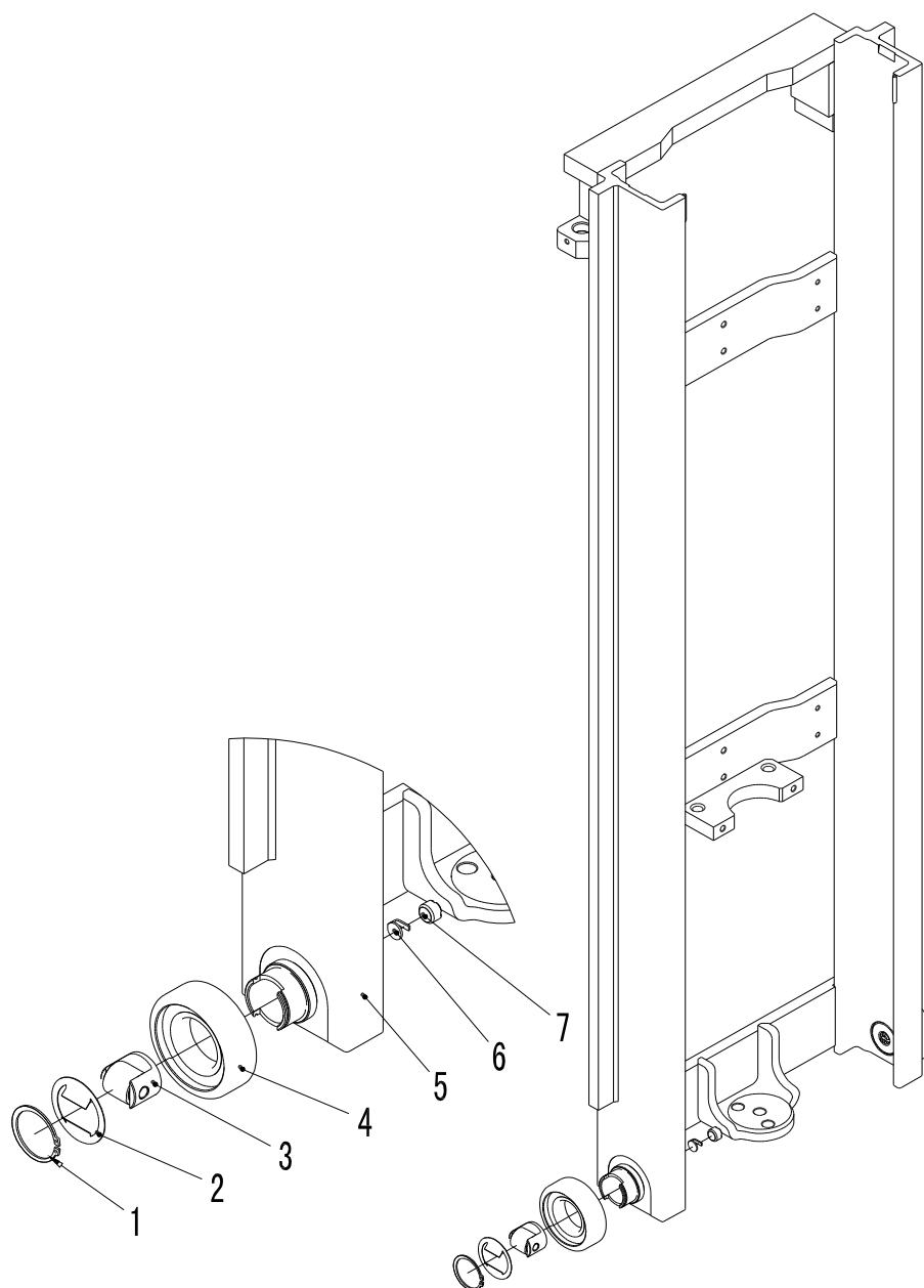
Рис. 102 Внутренняя мачта(СВМ1А-04001)
