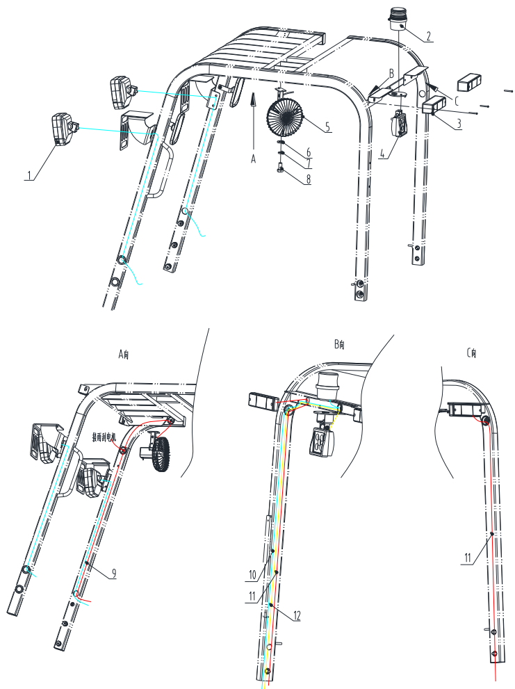
Рис. 53 Электрическая система CPD13, CPD16, CPD18, CPD20, CPD25
