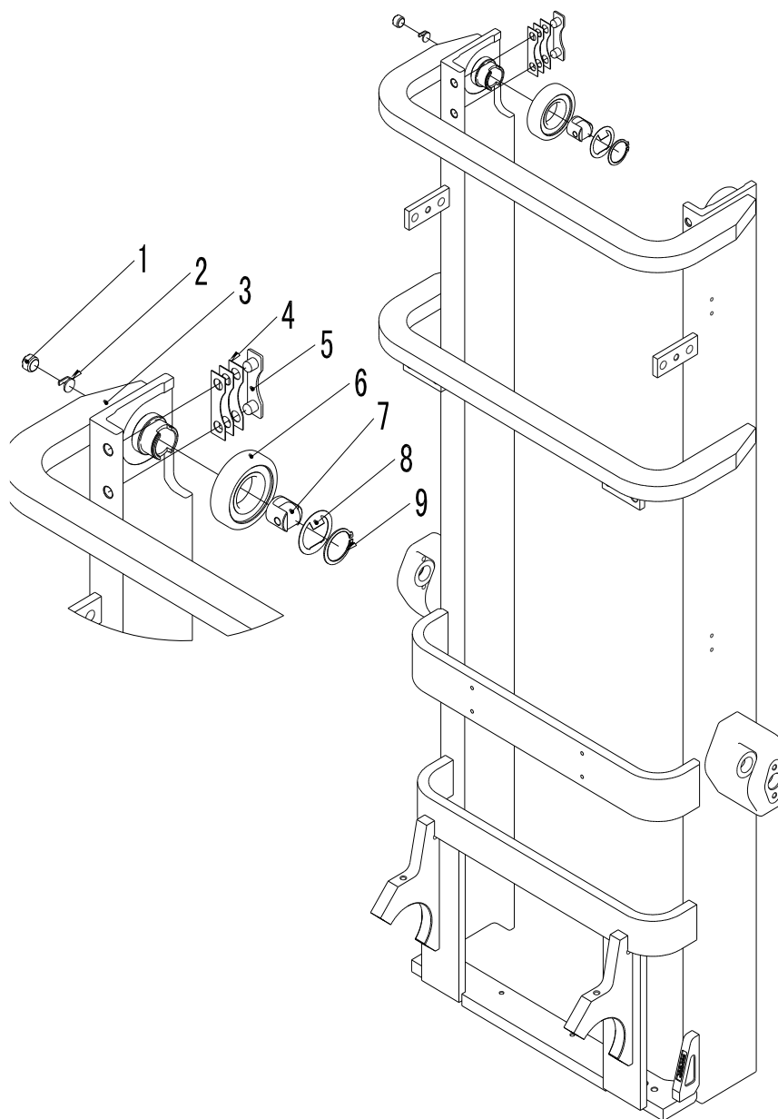
Рис. 101 Внешняя мачта (СВМ1А-02001)
