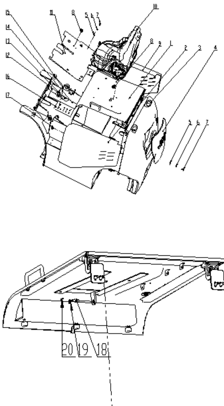
Рис. 21 Капот и панель пола CPD13, CPD16, CPD18, CPD20, CPD25
