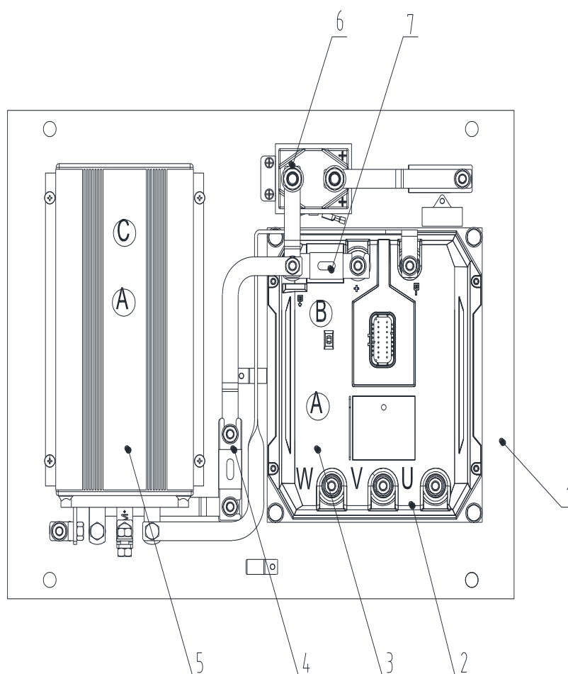
Рис. 38 Электрическая система CPD20, CPD25
