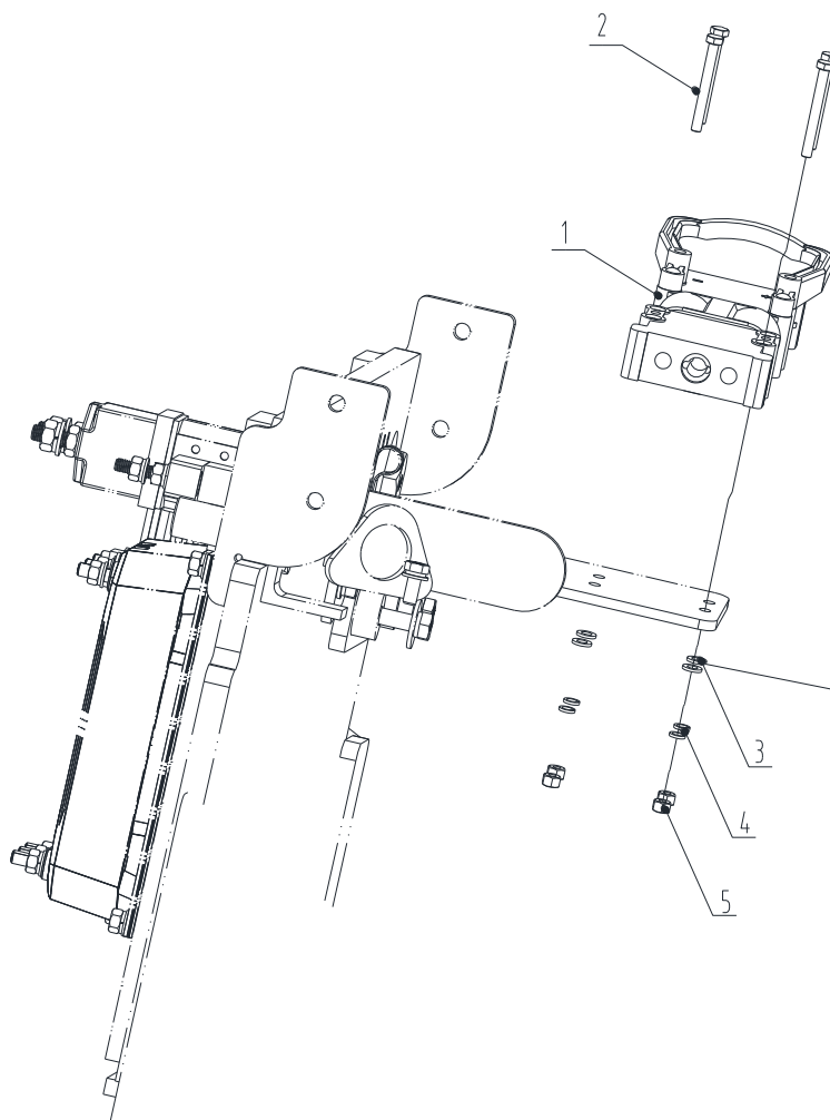
Рис. 52 Электрическая система CPD20, CPD25
