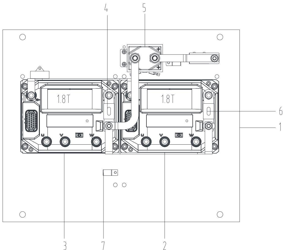
Рис. 35 Электрическая система CPD18
