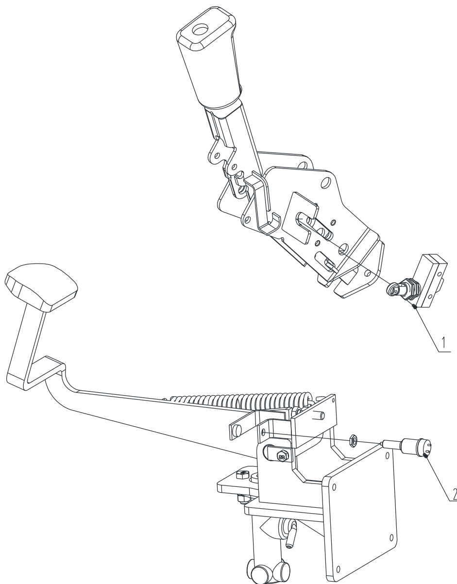
Рис. 55 Электрическая система CPD13, CPD16, CPD18, CPD20, CPD25
