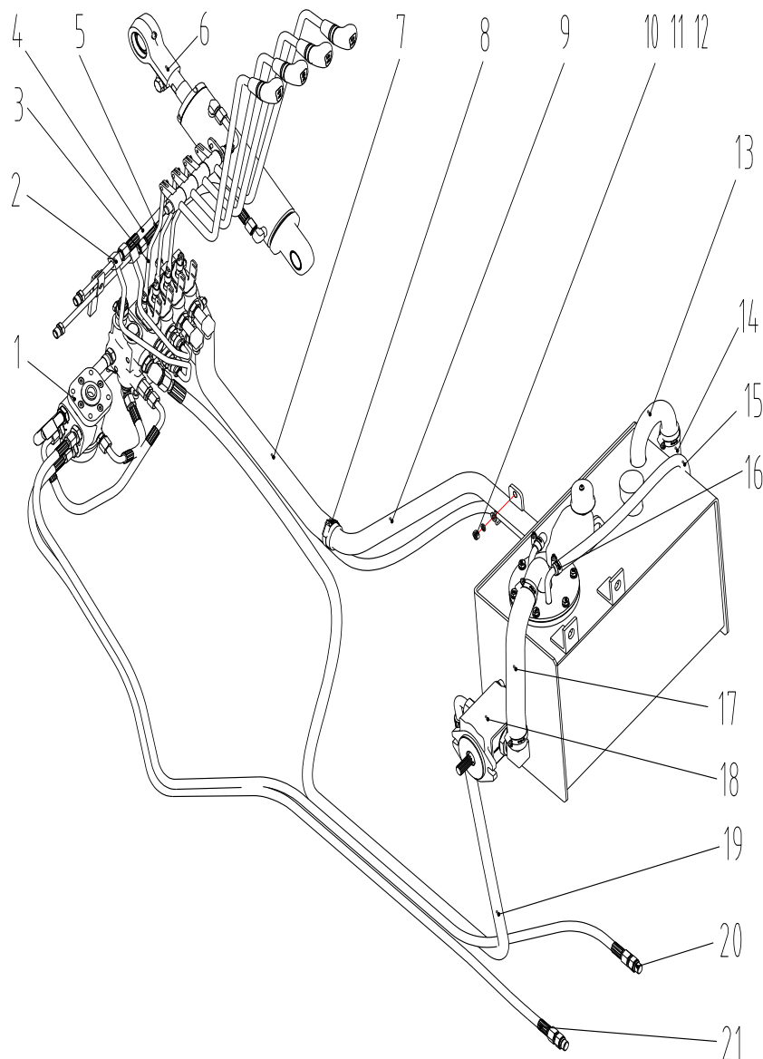
Рис. 90 Гидравлическая система CPD13, CPD16, CPD18/ CPD20, CPD25
