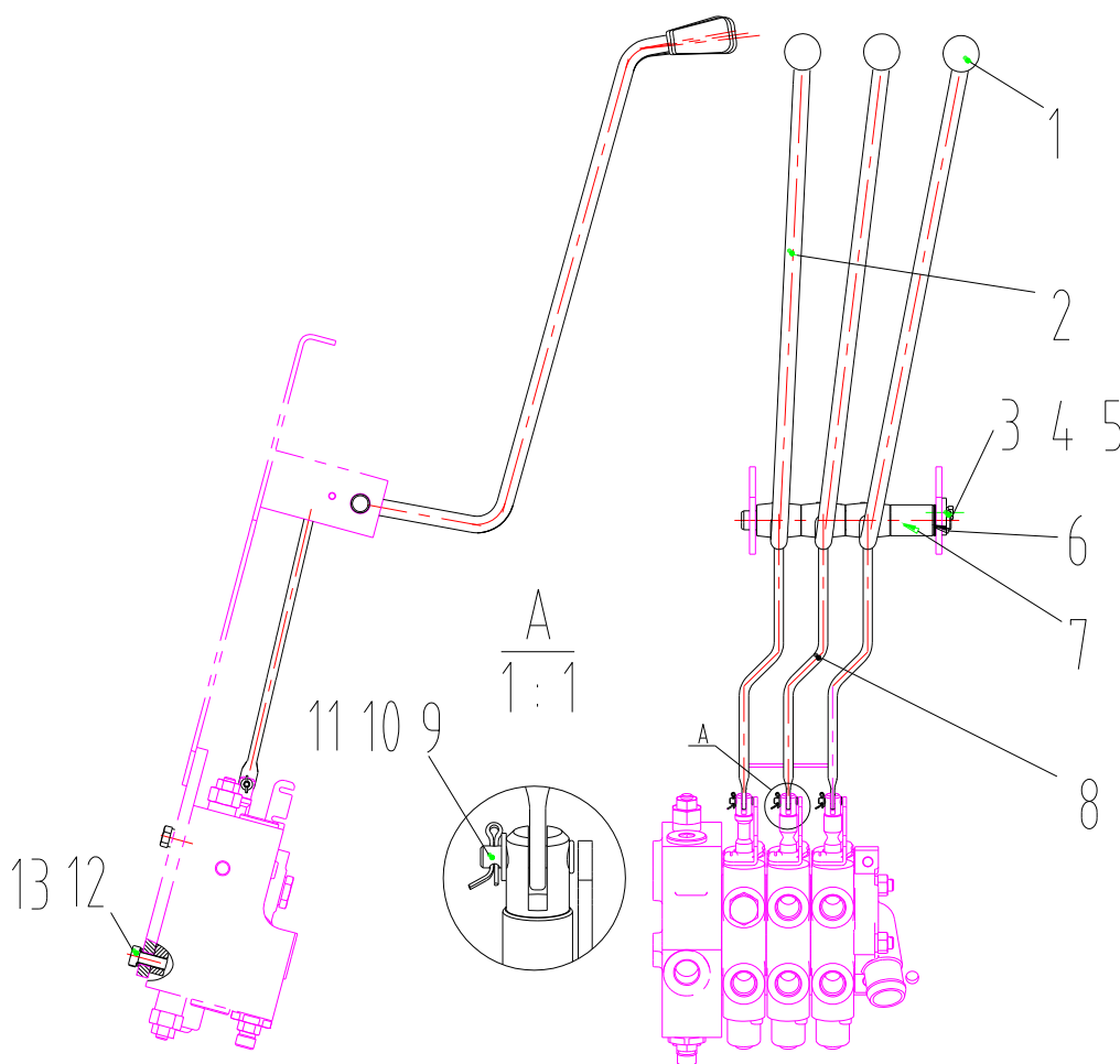
Рис. 94 Блок управления клапаном CPD13, CPD16, CPD18/ CPD20, CPD25
