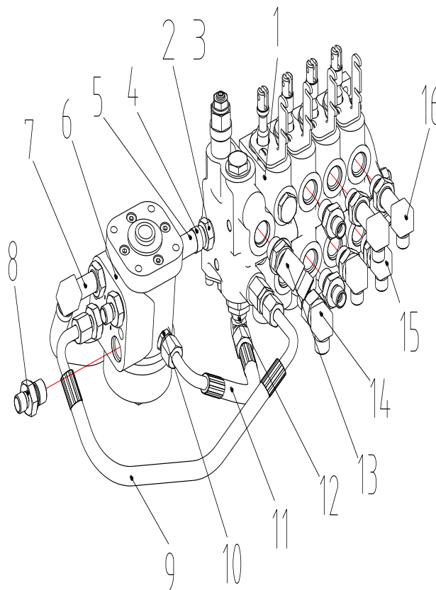
Рис. 91 Гидравлическая система CPD13, CPD16, CPD18/ CPD20, CPD25
