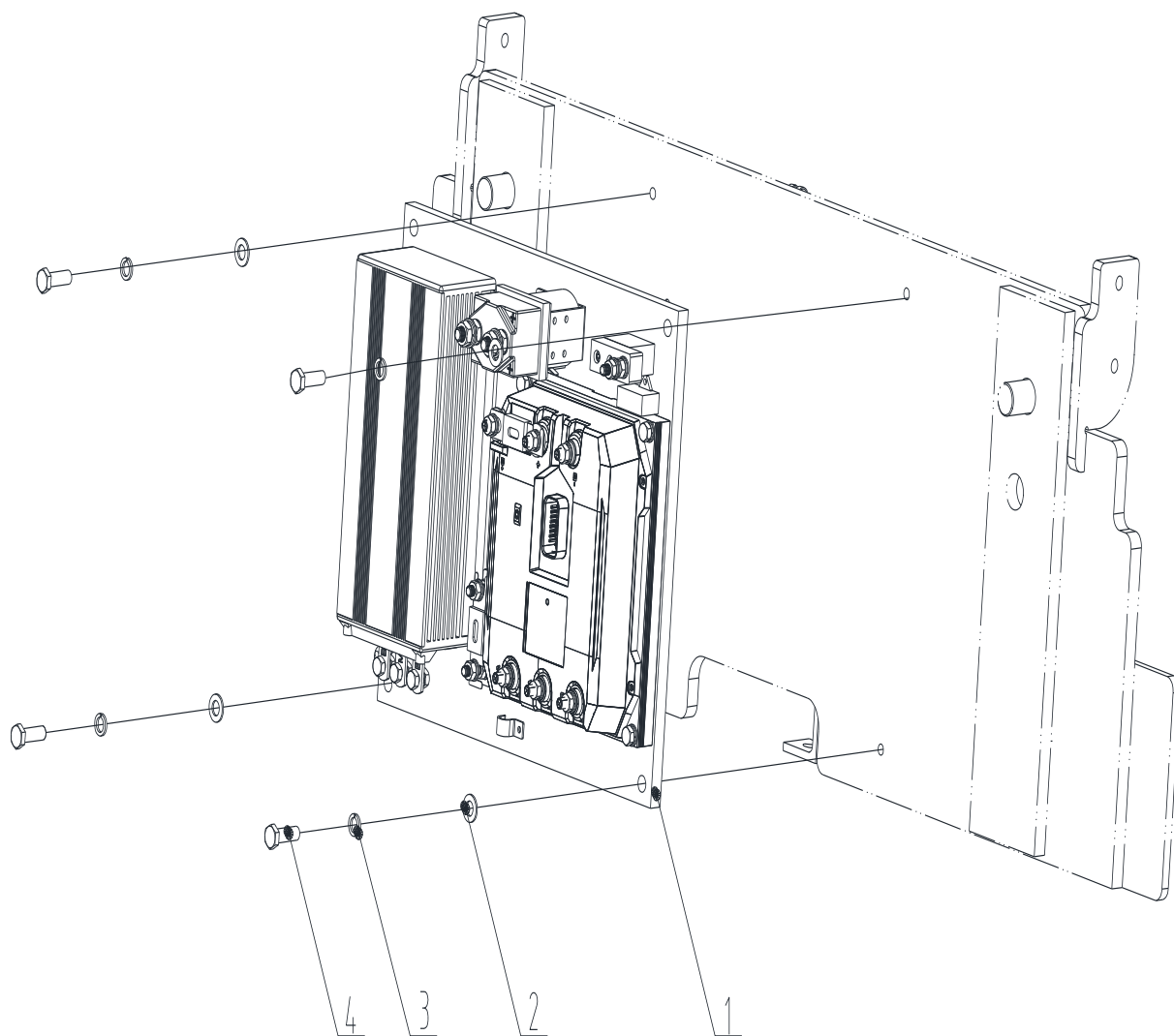
Рис. 69 Электрическая система CPD20, CPD25
