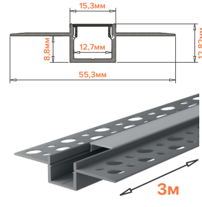
WAP-I-55/13/3000-A
