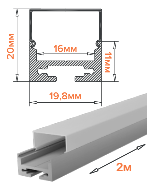
WAP-S/H-20/20/2000-A
