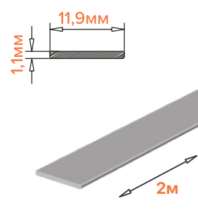
WAP-S-12/1/2000-A
