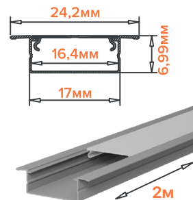
WAP-I-24/7/2000-A-LITE
