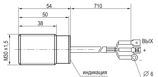
Габаритный чертеж
