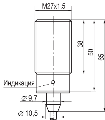
Габаритный чертеж
