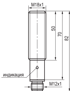
Габаритный чертеж
