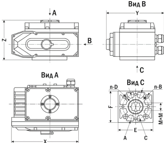
Габаритный чертёж
