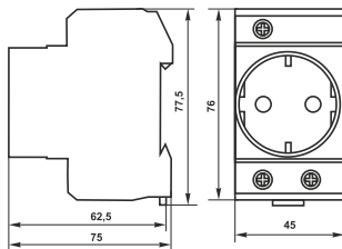
РДЕ-47
