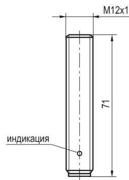
Габаритный чертеж
