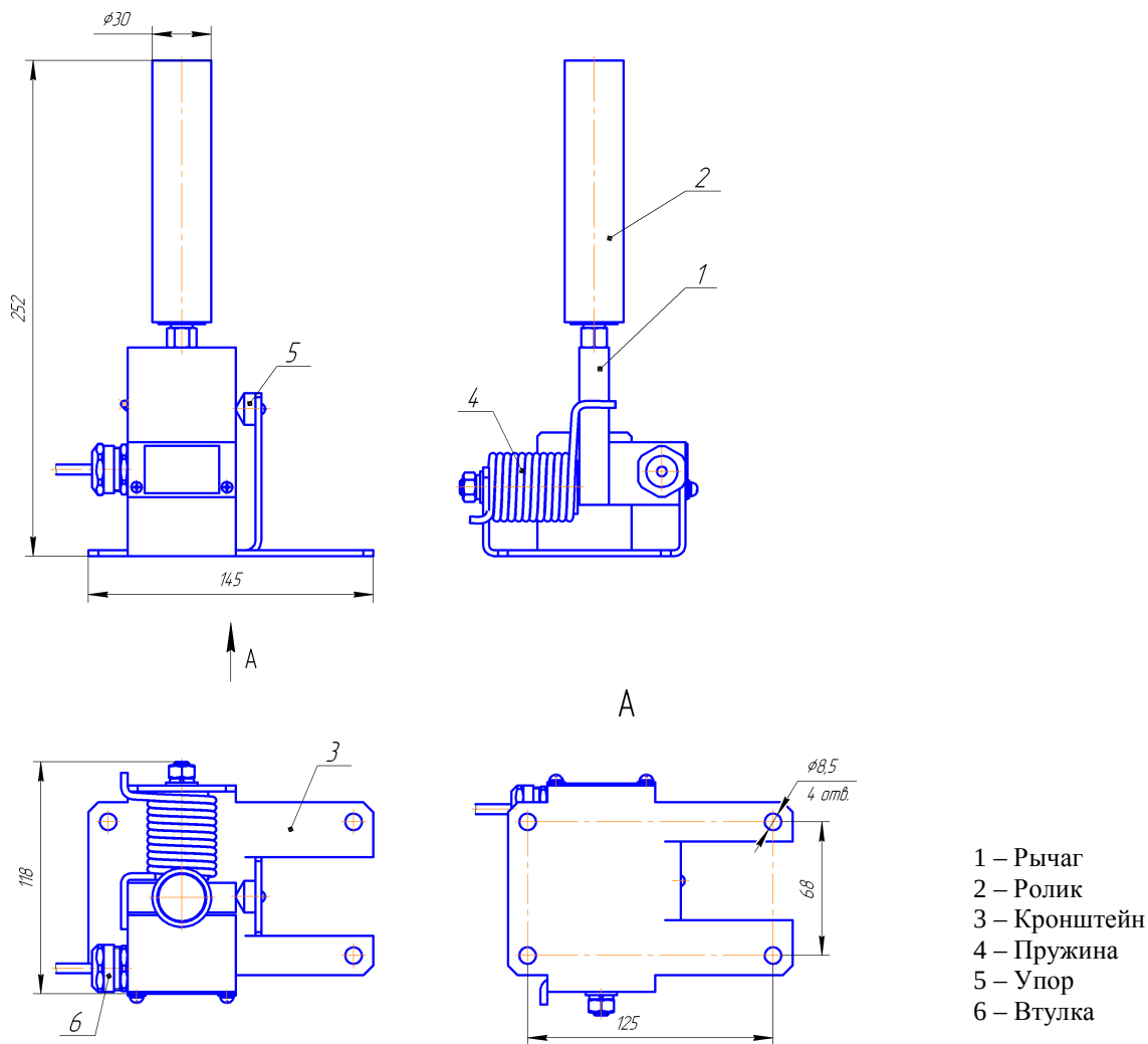
Рис.1. Габаритный чертёж датчика.
