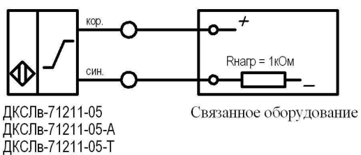
Рис.2. Схема подключения к оборудованию.
