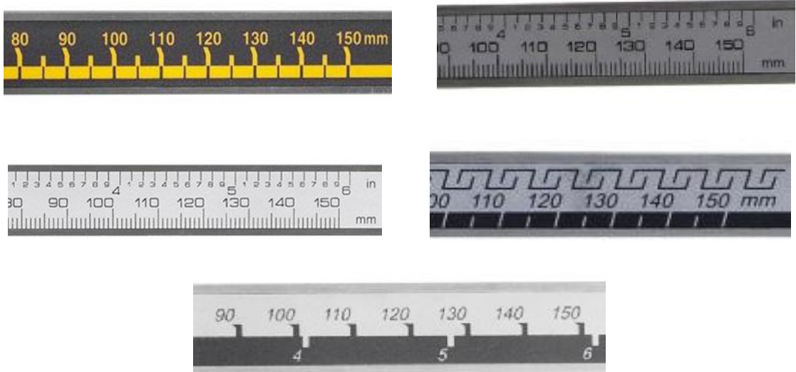
Рисунок 9 – Внешний вид штанги штангенциркулей ШЦЦ с оцифровкой
