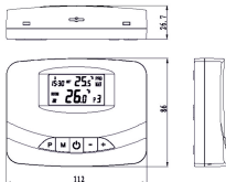
Термостат
