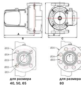
Рисунок 1 – Габаритные размеры
