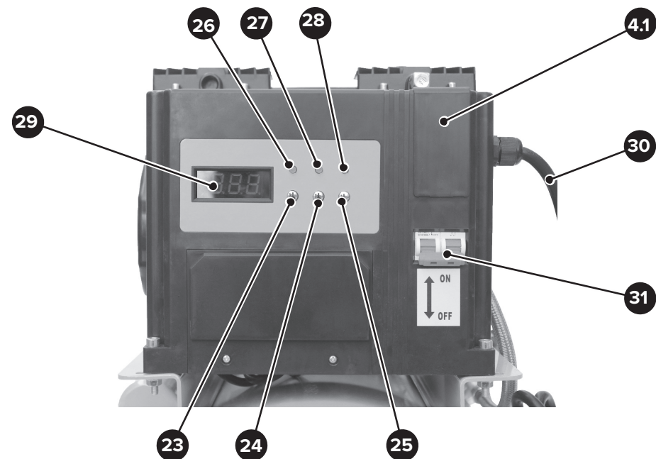
Рисунок 2. 3 — Блок управления и контроллер компрессора AC-720-100-OFHS
