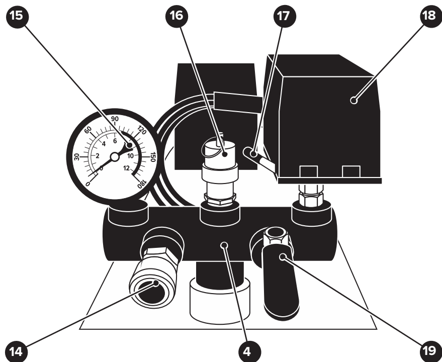
Рисунок 2.4 — Блок управления и узлы компрессора AC-450-100-OFS (ID 1124)
