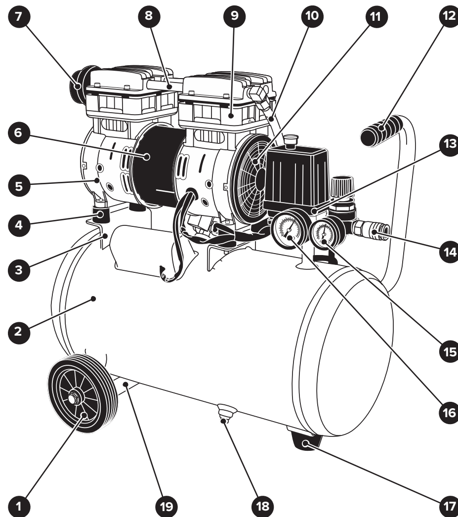
Рисунок 1.2 — Общий вид компрессора AC-180-24-OFS (ID 1124)
