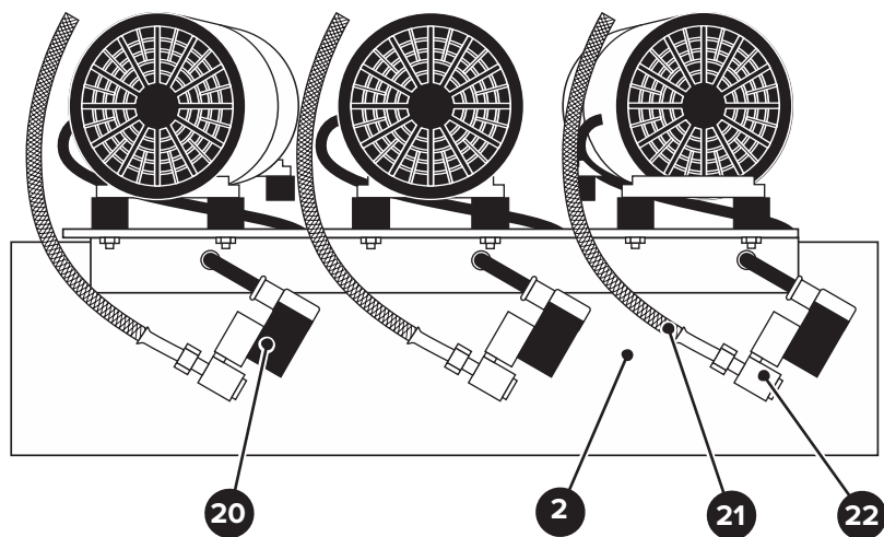
Рисунок 2.4 — Блок управления и узлы компрессора AC-450-100-OFS (ID 1124)
