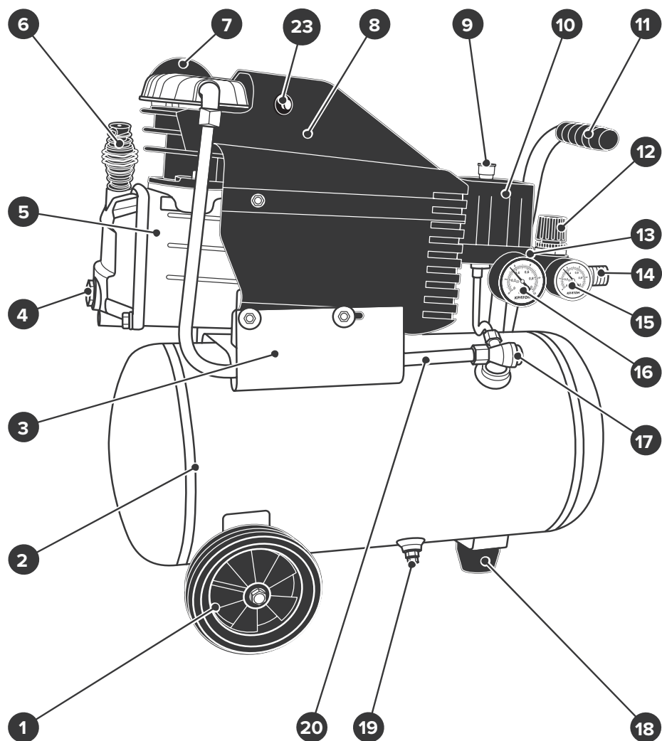
Рисунок 1.3 — Общий вид компрессора AC-210-24-DD (ID 1124), AC-260-24-DD (ID 1124), AC-280-40-DD (ID 1124)
