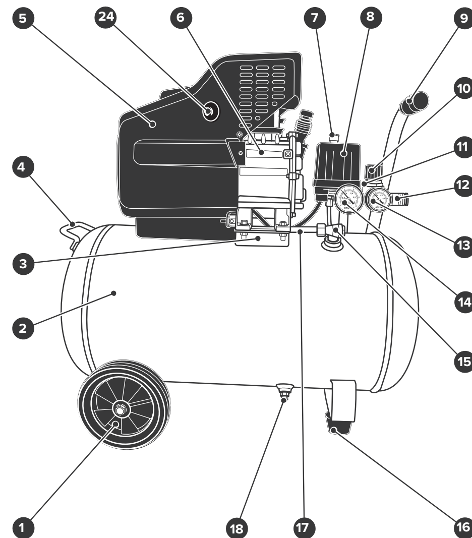
Рисунок 1.4 — Общий вид компрессора AC-300-40-DD (ID 1124)
