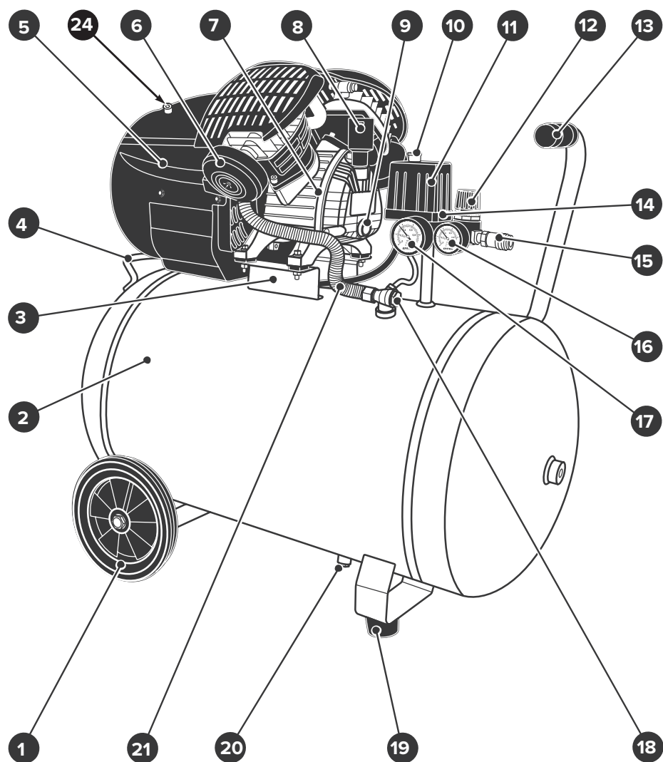
Рисунок 1.5 — Общий вид компрессора AC-350-50-DDV (ID 1124) , AC-360-100-DDV (ID 1124)
