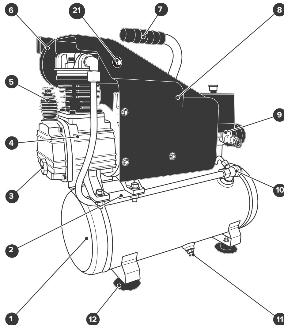
Рисунок 1.1 — Общий вид компрессора AC-175-6-DD (ID 1124)
