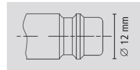
Вид штекера
