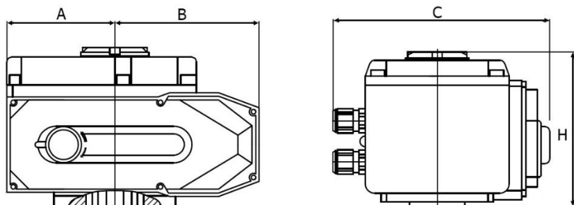
Рисунок 3 – Размеры электроприводов 100/150 Нм
