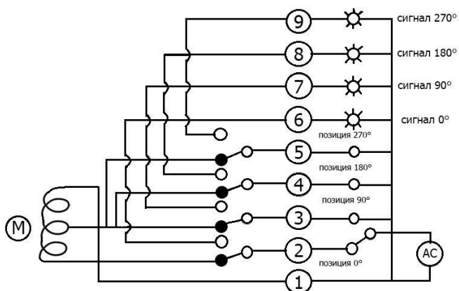
Рисунок 5 - Электросхема
