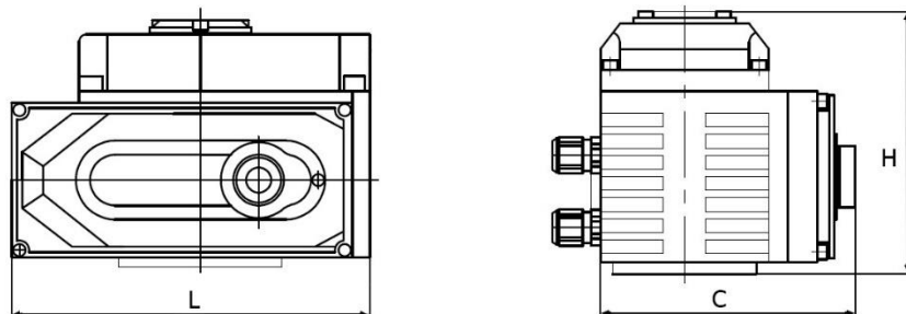
Рисунок 2 – Размеры электроприводов 50/80 Нм
