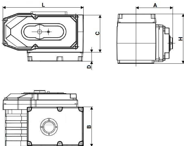
Рисунок 4 – Размеры электроприводов 200/600 Нм
