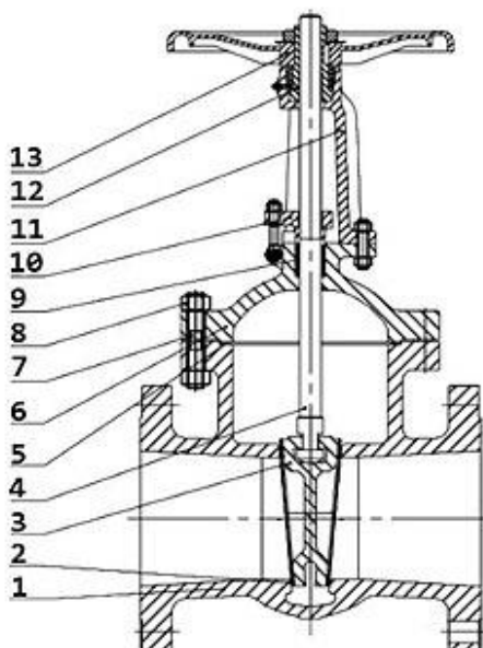
Рисунок 1- Деталировка
