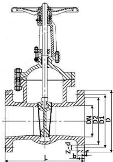
Рисунок 2 - Размеры
