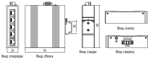
Рис. 1 — Габаритные размеры DASW-205
