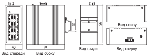
Рис. 1 — Габаритные размеры DASW-208
