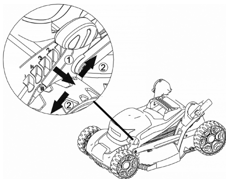
Рис. 11 Регулировка высоты скашивания
