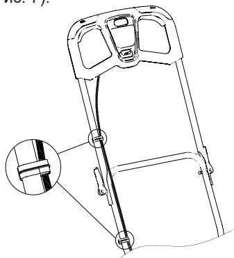
Рис. 7 Фиксация кабеля включения
