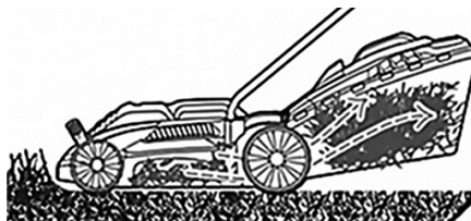
Рис. 2 Движение травы при скашивании
