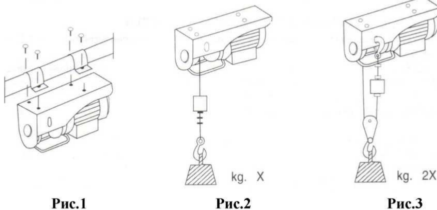
Рисунок 1. Установка мини тали.
