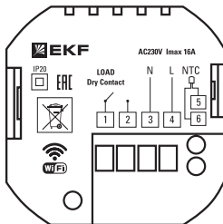
Рисунок 2 – Схема расположения клемм: 1,2 — нагрузка (бойлер); 3,4 — сеть; 5,6 — датчик
