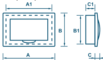
Рис. 1 – Встраиваемая установка
