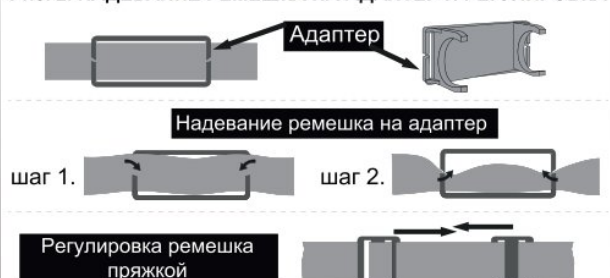
Рис. 2. НАДЕВАНИЕ РЕМЕШКА НА АДАПТЕР И РЕГУЛИРОВКА
