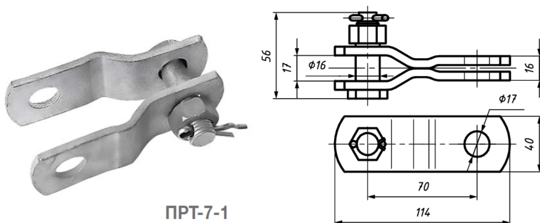
Рис. 1. Внешний вид промежуточного звена ПРТ-7-1.
