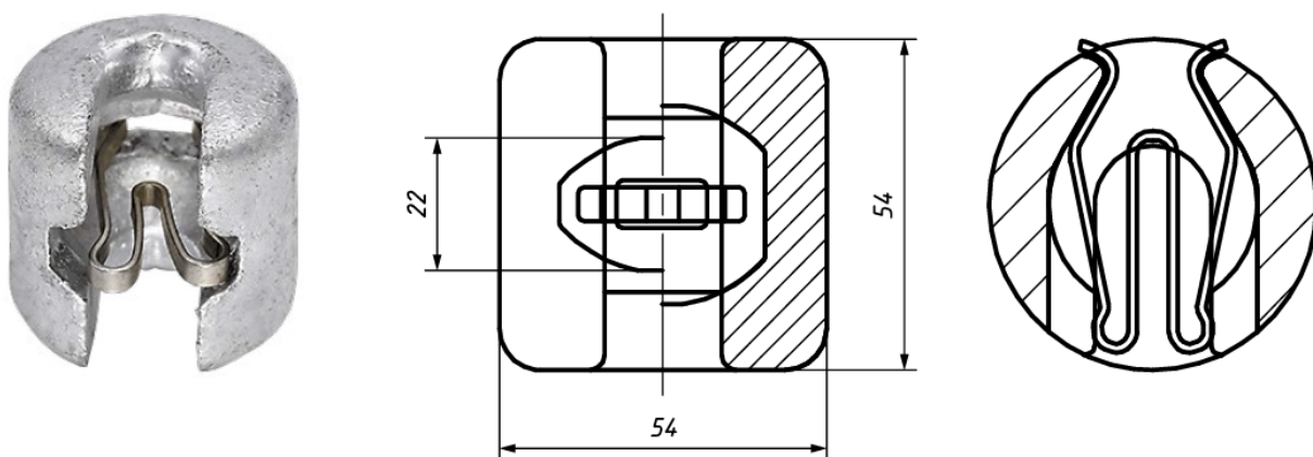
Рис. 1. Внешний вид ушка УД-7-16.
