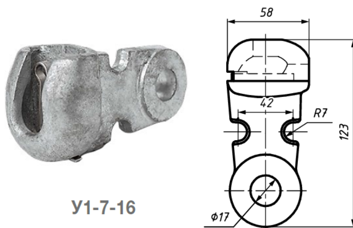
Рис. 1. Внешний вид ушка У1-7-16.
