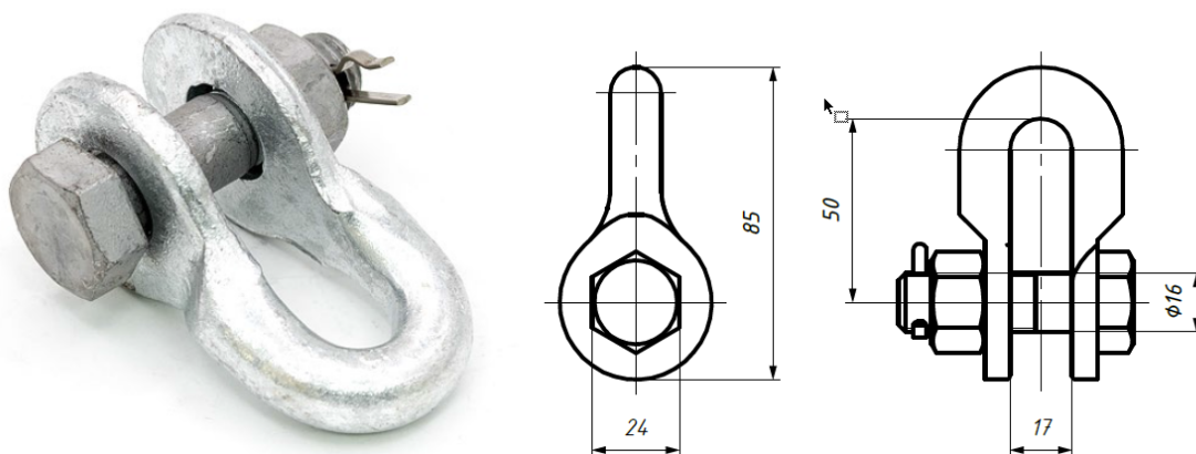
Рис. 1. Внешний вид скобы СК-7-1А.
