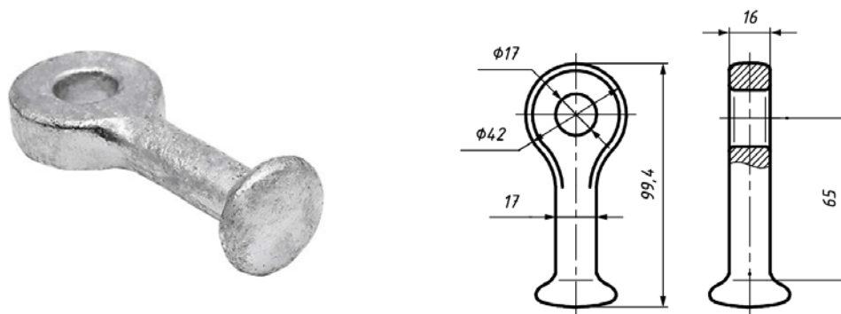
Рис. 1. Внешний вид серьги СР 7-16.
