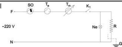
Figure 3: Contrôle Manuel du Correcteur Panneau Electrique Schéma électrique
