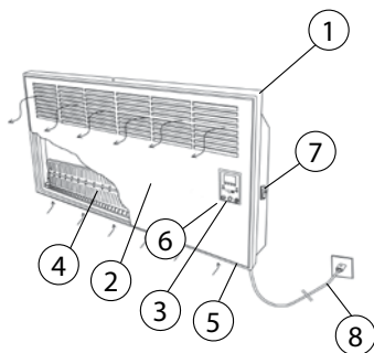
2. ábra: Digitális konvektor teljes kép
