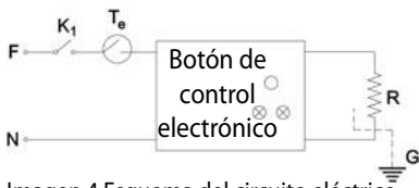
Imagen 4 Esquema del circuito eléctrico del convector panel con unidad de control electrónico
