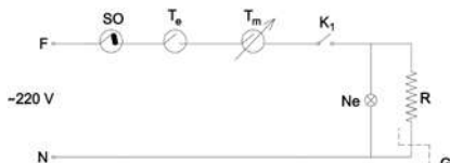
Slika 3: Šema Strujnog Kola Panelnog Konvektora sa Manualnom (Ručnom) Kontrolom
