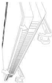
Figura 8. Posizionare il Termoconvettore sul gancio inferiore
