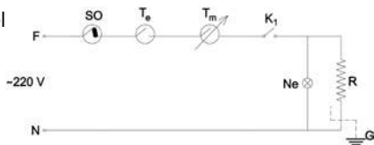
3. ábra: Mechanikus panel konvektor fűtés
