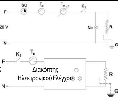
Σχήμα 4. Διάγραμμα Ηλεκτρικού Κυκλώματος του Επίπεδου (Ψηφιακού) Θερμοπομπού
