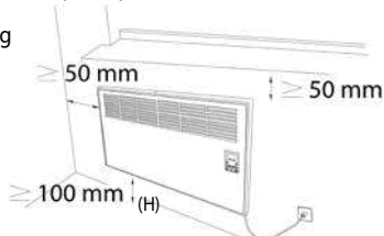
Slika 6: Minimalne sigurnosne zone potrebna za efikasnost uređaja
