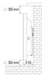
Bild 11. Abmessungen der Standheizkörper in montierter Stellung
