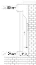
Figura 11. Dimensões montadas do convetor
