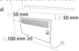
Bild 6. Mindestabstände für eine effiziente Funktionstüchtigkeit des Gerätes
