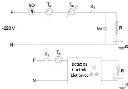
Figura 4. Diagrama do Circuito Elétrico do Convector de Painei com Unidade de Controle Digital
