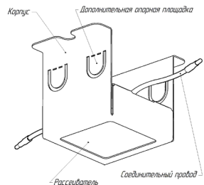
Рисунок 1в – основные части светового модуля Tetrис
