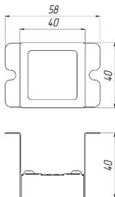
Рисунок 1а – габариты светового модуля Tetrис
