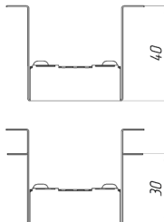
Рисунок 1б – установочная глубина модуля в вариантах с отогнутыми дополнительными опорными площадками и без
