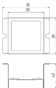
Рисунок 1а – габариты светового модуля Tetrис
