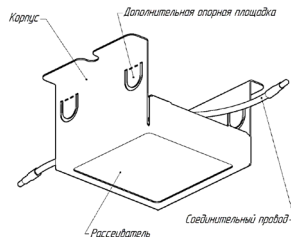
Рисунок 1в – основные части светового модуля Tetrис
