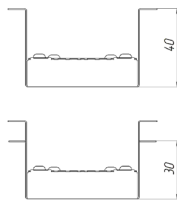
Рисунок 1б – установочная глубина модуля в вариантах с отогнутыми дополнительными опорными площадками и без
