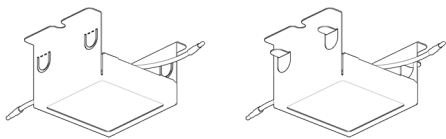
Рисунок 6 – Отгибание опорных площадок для установки светильника в потолок с высотой ламели 30мм.
