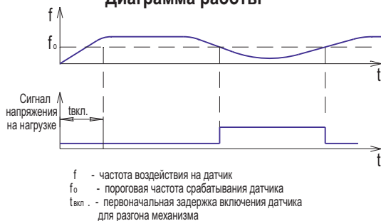
Диаграмма работы
