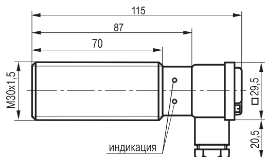
Габаритный чертеж
