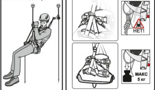
Рис. 13. Пример организации системы канатного доступа
