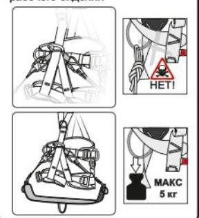
Рис. 14. Способ интеграции рабочего сидения
