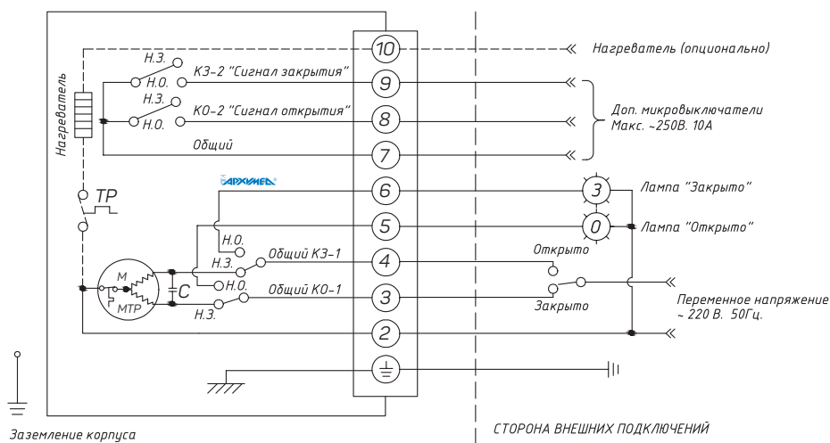
Схема подключения электропривода
