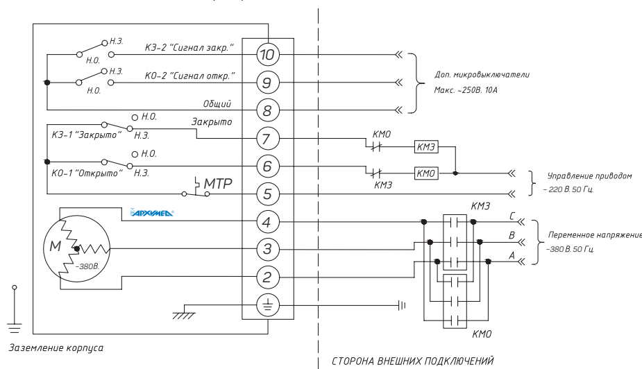
Схема подключения электропривода
