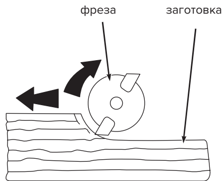
Рисунок 6 — Правильно выбранное направление движения подачи фрезера относительно направления вращения фрезы.
