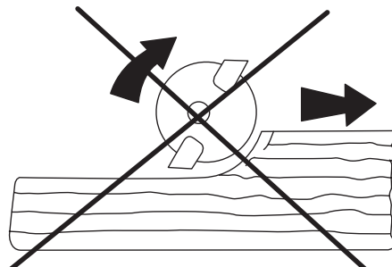
Рисунок 6 — Неверно выбранное направление движения подачи фрезера относительно направления вращения фрезы.
