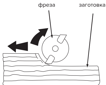
Рисунок 5 — Правильно выбранное направление движения подачи фрезера относительно направления вращения фрезы.
