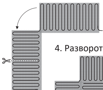
3. Разворот части на 90° и второй разрез сетки мата.
